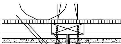
Samleprofil 1:5
