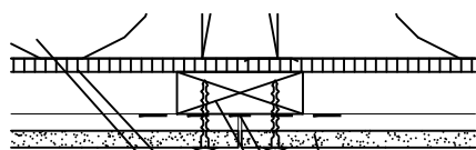
Stødsamling 1:5
