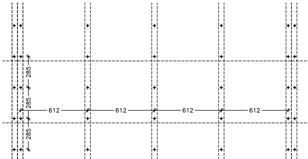
Opstalt af en Cedral Board 1:20
